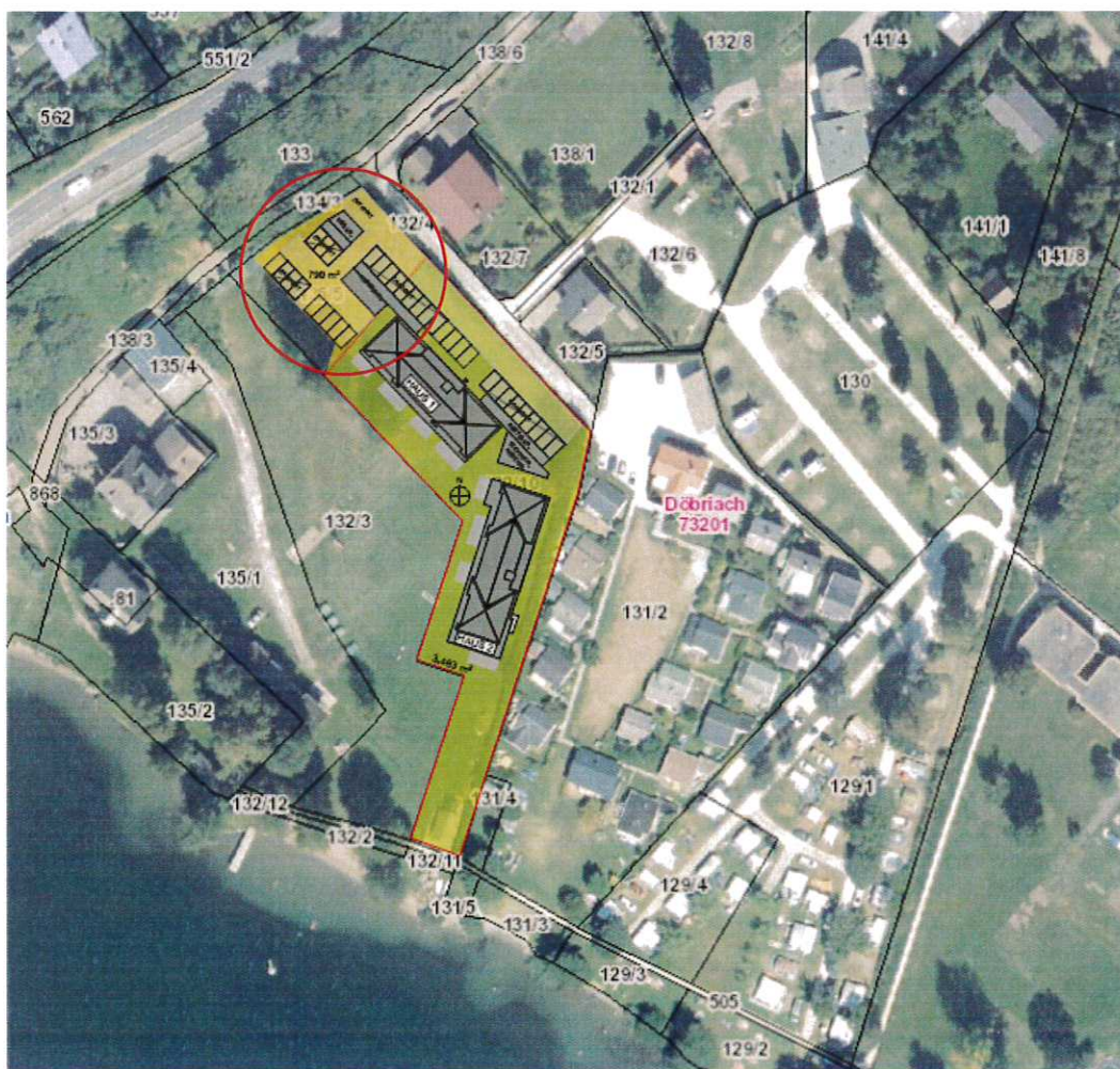
LAGEPLAN 1:1000
